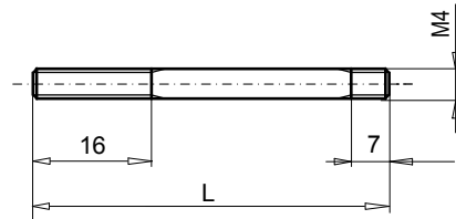
STIFTSCHRAUBE M4xL
