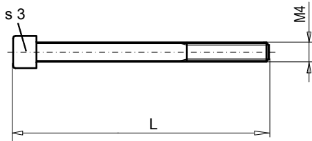
ZYLINDERSCHRAUBE M4xL
