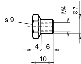
HALSMUTTER M4
