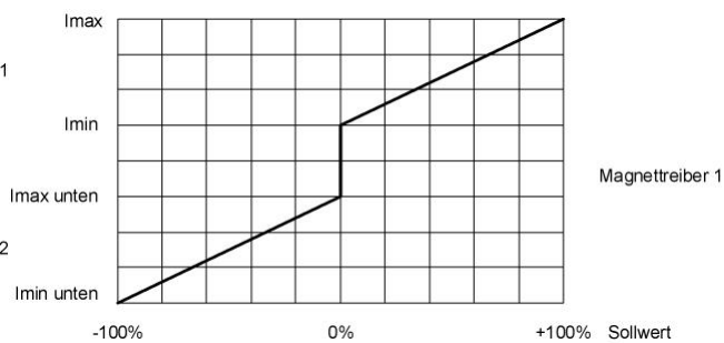
4/3-Wege 1-Magnet
